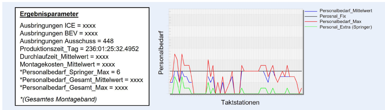
Bild 5. Analyse des minimalen und maximalen Personalbedarfs sowie zusätzlich benötigter Personen (Springer) für das Verteilszenario 10% BEV (battery electric vehicle)- und 90% ICE (internal combustion engine)-Typenvertreter. Grafik: Hörmann Rawema
