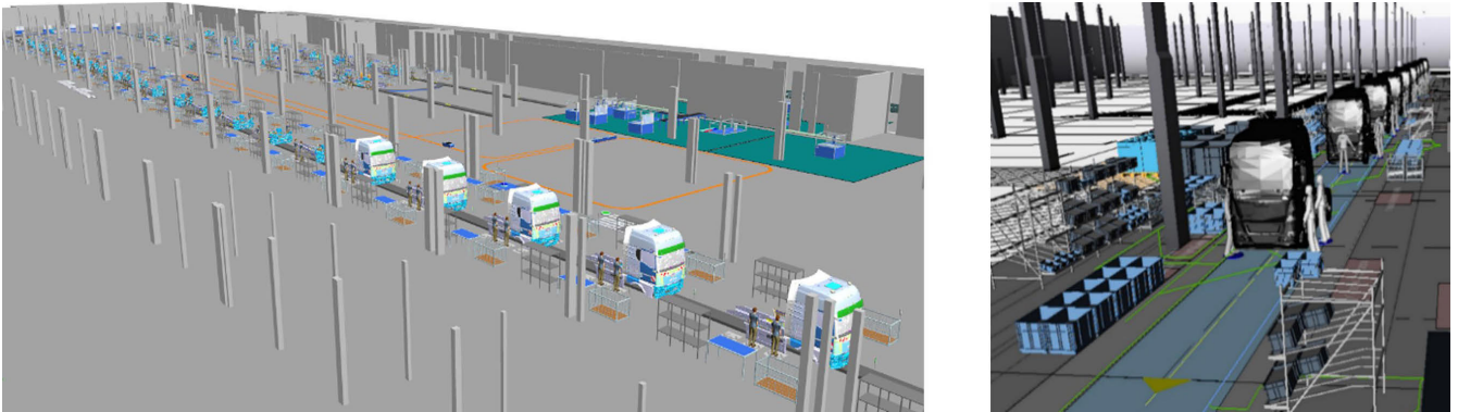
Bild 4. Links: Simulationsmodell der Montagelinie auf Makroebene. Rechts: Simulationsmodell ausgewählter Stationen auf Mikroebene. Grafik: Hörmann Rawema (links), Fraunhofer IGCV (rechts)
