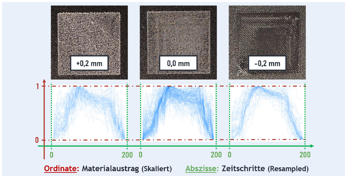
Bild 5. Einschichtige Referenzbauteile bei variablem Offset der Austrageinheit (oben). Verlauf des Materialaustrags beim Herstellen der Referenzbauteile (unten). Skalierung des Materialaustrags auf den Wertebereich [0,1] sowie Resampling der Abtastung auf 200 Werte. Grafik: wbk
