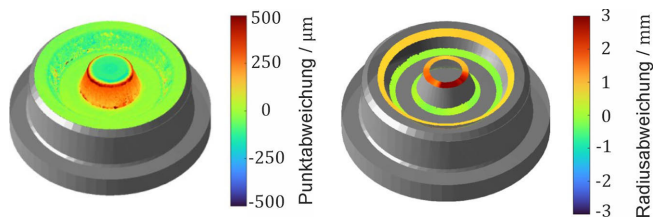
Bild 5. Punkt- und Merkmalsabweichungen am Obergesenk des Demonstratorwerkzeugs. Grafik: IMR
