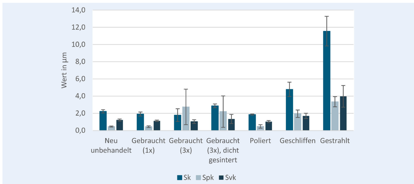
Bild 5. Rauheitskennwerte Sk, Spk und Svk der analysierten Sinterunterlagen. Grafik: Fraunhofer IAPT
