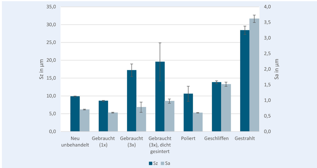
Bild 4. Rauheitskennwerte Sz und Sa der analysierten Sinterunterlagen. Grafik: Fraunhofer IAPT
