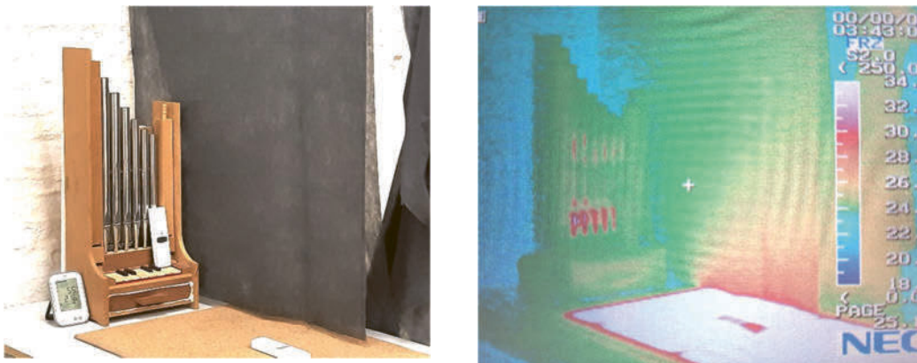
Abb. 1 Aufbau Orgel hinter Teppich mit Thermographiebild
