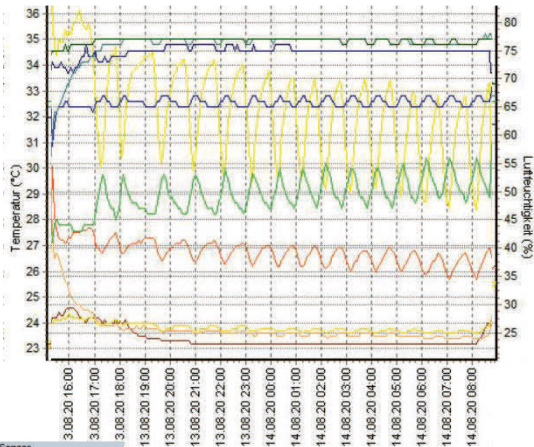
Abb. 19 Klimadaten
